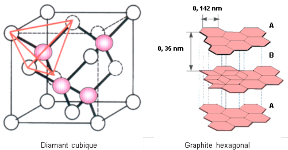
Figure 2 : Structures cristallographiques à température ambiante.
