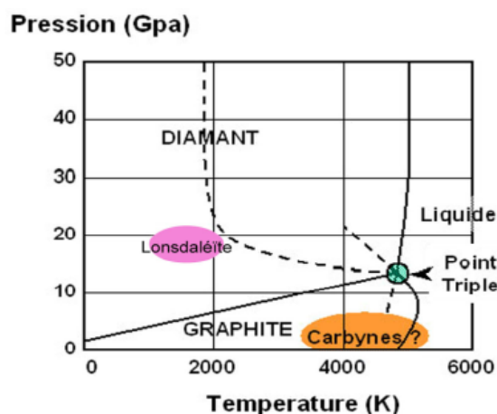
Figure 1 : Diagramme de phases du carbone
