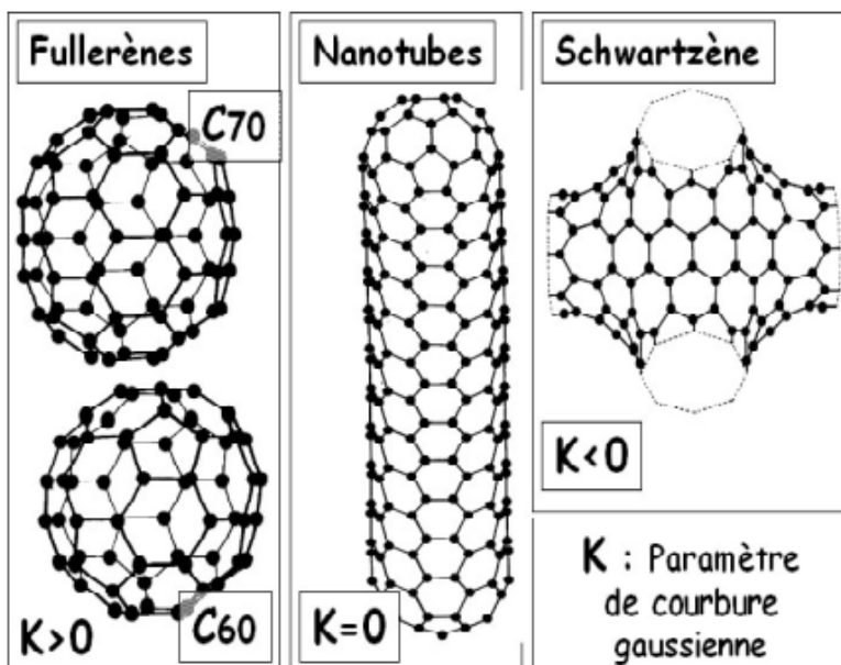
Figure 3 : Structures tri-coordonnées sur des surfaces courbes
