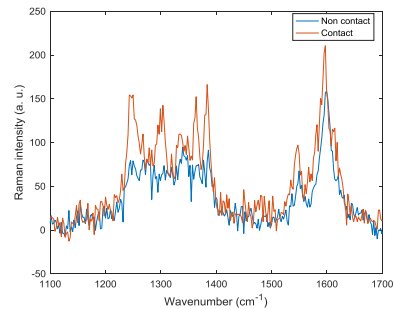
Figure 3 : spectre Raman singulier fortement dépendant de la position de la pointe Ag.
