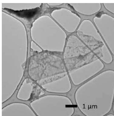
Figure 1 : Image MET d'un feuillet de graphène issue d'un GIC de FeCl_3 agité pendant 6 jours dans du toluène.
