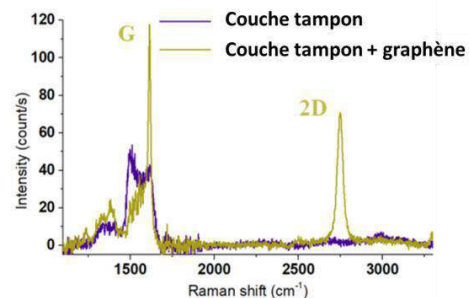
Figure 2 : Exemples de spectre Raman de la couche tampon seule (violet) et de la couche tampon recouverte d'une monocouche de graphène (vert).
