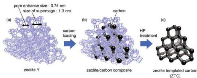
Figure 1 : Schéma de la méthode de fabrication de la zeolite-templated carbon (ZTC) [3]
