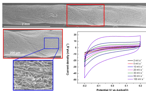
Figure 1 : Images MEB d'une tresse de nanofibres de lignine et ses propriétés électrochimiques résultantes après pyrolyse à 1000°C.
