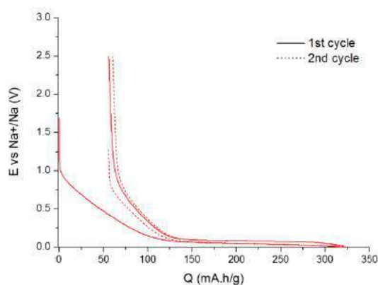
Figure 1: Premiers cycle galvanostatique avec un carbone dur issu d'un mélange de brai et de lignine. Demi-pile bouton vs. Na + /Na à un régime de courant de C/20.
