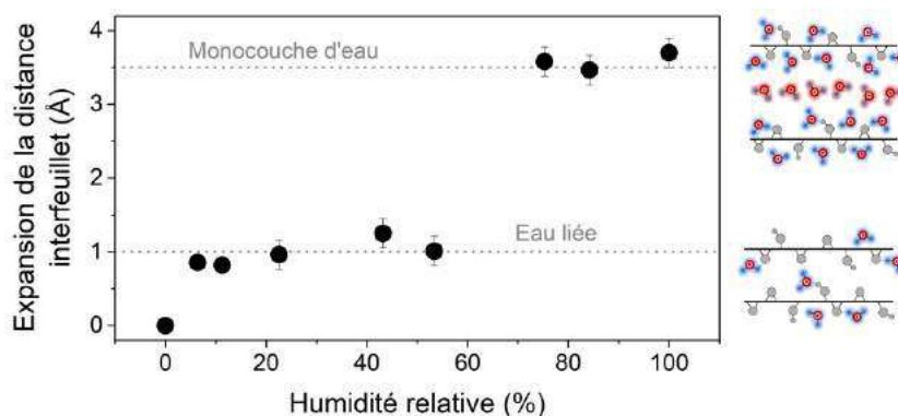
Figure : Expansion de la distance interfeuille à l'équilibre, en fonction de l'humidité relative et représentation schématique du phénomène d'hydratation (les atomes d'oxygène et d'hydrogène des molécules d'eau sont représentés en rouge et en bleu).
