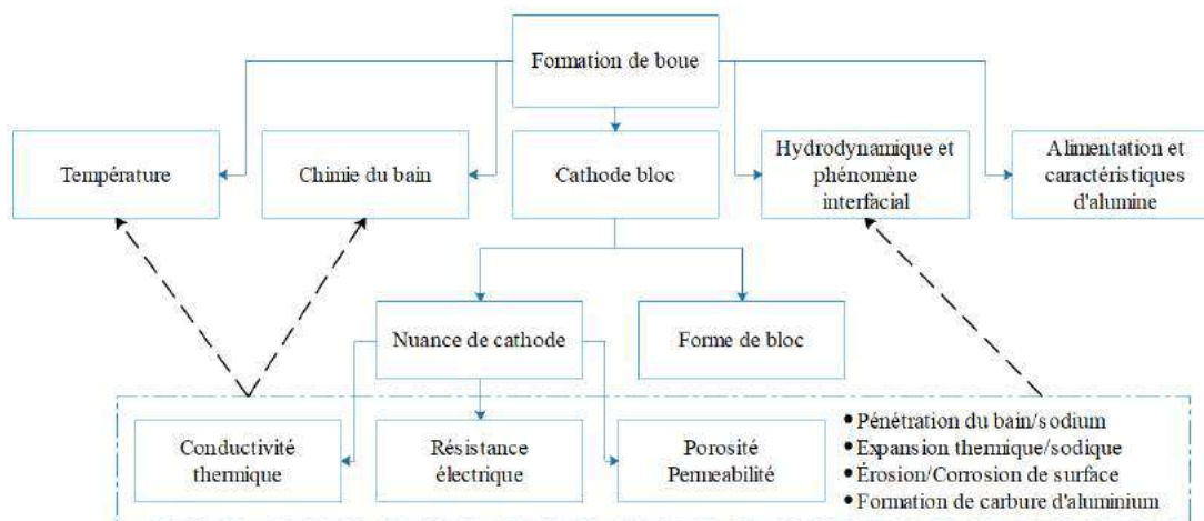
Figure 1 : Les facteurs importants concernant la formation de boue dans le procédé Hall-Héroult
