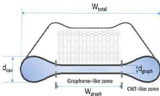
Figure 1: Image schématique de nanotube de carbone aplatis dit dogbone, obtenu par la combinaison de une nanoruban de bi-graphène et deux cavités similaires aux tubes circulaires.
