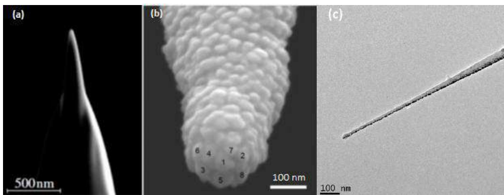
Figure 1 : (a) Image SEM d'une pointe TERS en argent [2] (b) Image SEM d'une pointe TERS recouverte d'or [3] (c) Image TEM d'une pointe nanocône de carbone recouverte d'or.
