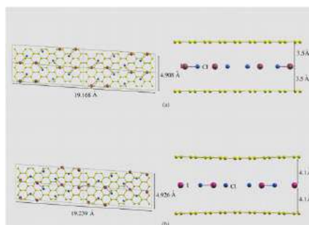
Figure 1 Représentation schématique de l'intercalation de la molécule ICl entre les couches de graphène
