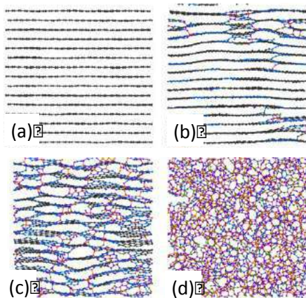
Figure 1: Modèles atomistiques de graphite (a) vierge, irradié à (b) 0.2 dpa, (c) 1 dpa et (d) amorphisé. (b) et (c) sont tirés de [1].
