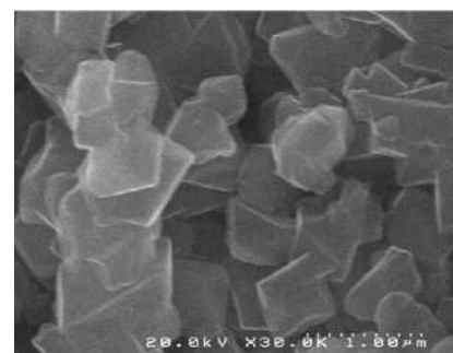
Figure 2 : Image obtenue au MEB après dissolution de la zéolite à l'acide fluorhydrique
