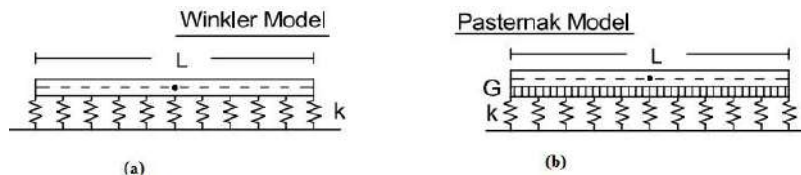
Fig. 1 les modèle du milieu élastique : (a) modèle Winkler, (b) Modèle Pasternak
