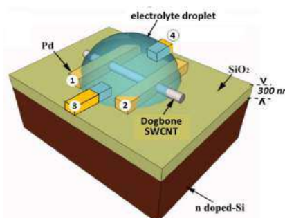
Figure 2 : Concept du transistor (CNTFET). Source (1), drain (2) et deux grilles latérales (3) et (4). Les grilles latérales fonctionnent aussi comme électrodes pour effectuer le remplissage asymétrique.
