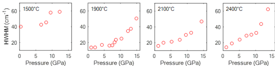
Figure 1 : Evolution de la largeur de la bande G en fonction de la pression pour différentes températures de recuit
