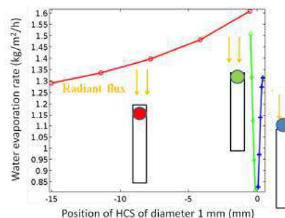
Figure 2 : Vitesse d'évaporation de l'eau de mer couverte d'une monocouche de sphères de carbone creuses de 1 mm de diamètre, calculée sous flux solaire de 1 \text{ kW/m}^2 en fonction de leur flottabilité.
