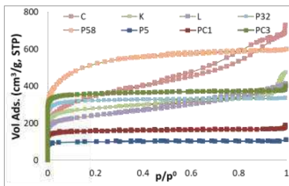
Figure 1 : Isothermes d'adsorption-désorption d'azote à 77 K des carbones nanoporeux sélectionnés dans cet étude.
