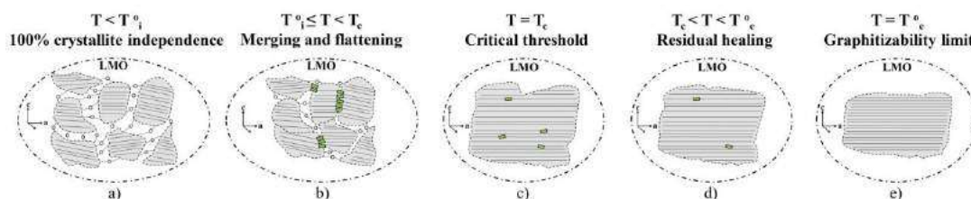
Figure 1 : Mécanisme topologique proposé pour la graphitisation des LMOs des carbones graphitables et non-graphitables opérant entre T_i (1700 K) et T_e (3400 K).
