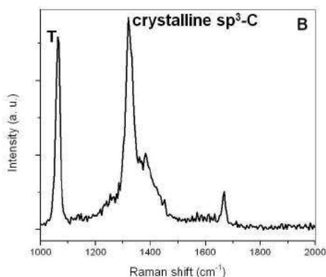
Figure 1 : Spectre Raman de quelques couches de graphène, obtenu après leur exposition au procédé d'hydrogénation par filaments chauds (excitation à 244 nm).
