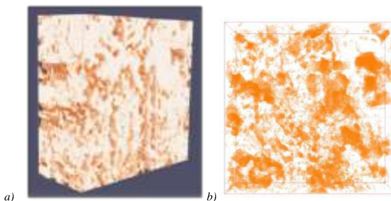
Figure 1 : a) reconstruction 3D d'un volume de 244 \times 244 \times 105 \text{ nm}^3 d'une matrice carbonée générant des hydrocarbures ; b) visualisation du réseau poreux de la matrice carbonée.
