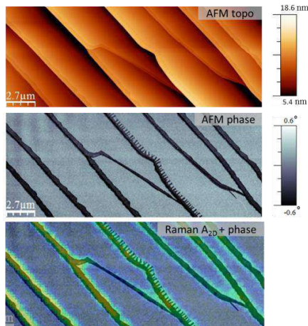
Figure 1 : Images AFM en mode topographie et phase et cartographie Raman de l'intensité intégrée de la bande 2D superposée à l'image AFM en mode phase réalisées sur une même zone d'un échantillon présentant les premiers instants de croissance du graphène en bord de marche.
