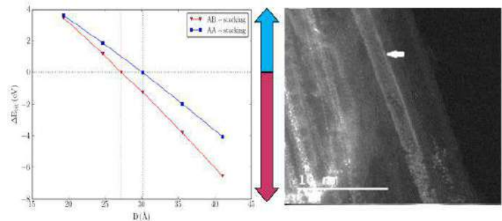
Figure 2 : DFT calcul du diamètre des nanotubes de carbone rempli avec une séquence équidistante de I 3 pour collapse stablement (gauche). ADF image expérimentale d'un nanotube avec dans I collapse (droite) [4].
