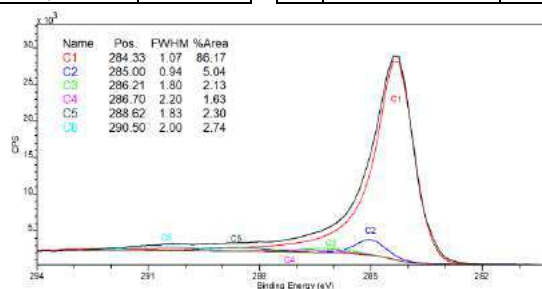
Figure 2 - Déconvolution du pic de coeur C1s avec identification des domaines associés à chaque région pour le rCB de vapo-thermolyse
