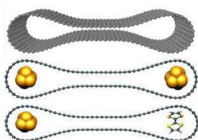
Figure 1 : nanorubans de bi-graphènes, préparés à partir de nanotubes de carbone mono-parois de diamètre large. La figure montre les nanorubans avec les bords vides, remplis symétriquement et remplis asymétriquement.
