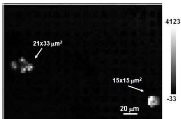
Figure 2 : Cartographie Raman (excitation à 244 nm) de l'intensité du mode d'élongation du diamant/lonsdaleite de quelques couches de graphène exposées au procédé d'hydrogénation par filaments chauds.
