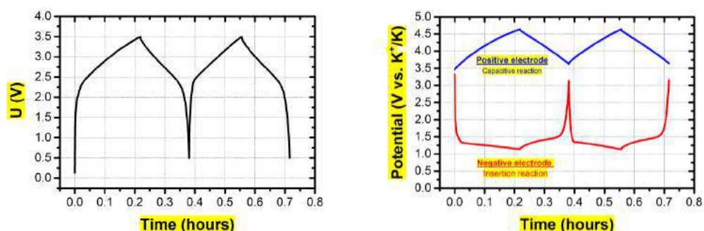
Figure 1: Profil de charge/décharge galvanostatique du supercondensateur hybride dans une configuration de cellules à trois électrodes. La tension de la cellule est imposée (noir) tandis qu'une électrode de référence permet de suivre le potentiel des électrodes positive (bleu) et négative (rouge).
