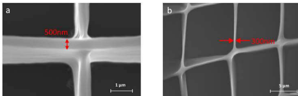
Figure 1 : Images MEB de microstructures réalisées par polymérisation multi-photons avant (a) et après (b) carbonisation
