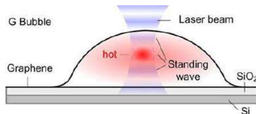
Figure 1 : Schéma de la bulle de graphène sur substrat interférentiel à onde stationnaire optique. Les points rouges indiquent où la bulle est la plus chauffée.
