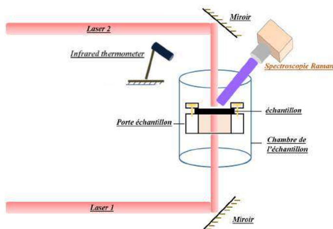
Figure 1 : Système de chauffage avec suivi in situ par spectroscopie Raman
